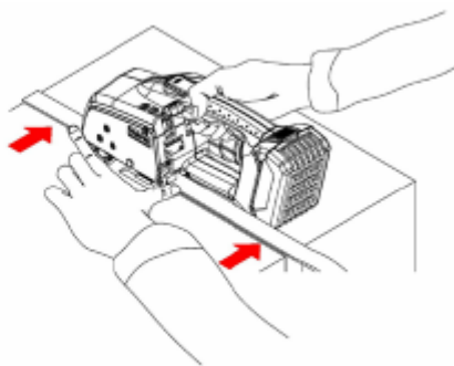
РИСУНОК 11. Протолкните ленты до упора
